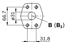
Вид Y
