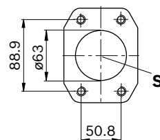
Вид X
